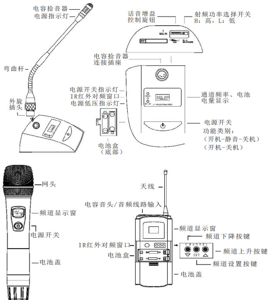
【图 5.1 无线发射端操作】
